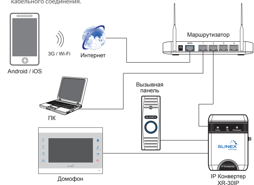
Схема 2. Подключение конвертера XR-30IP к сетевому интерфейсу посредством кабельного соединения.
